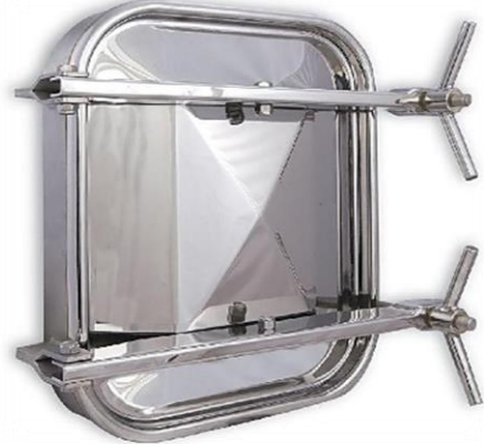
PORTELLA DA D=300mm A D=500mm
