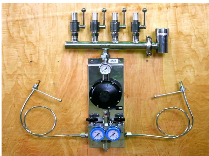
DISTRIBUTORI AZOTO/ARGON DA 2 A 10 UTENZE
